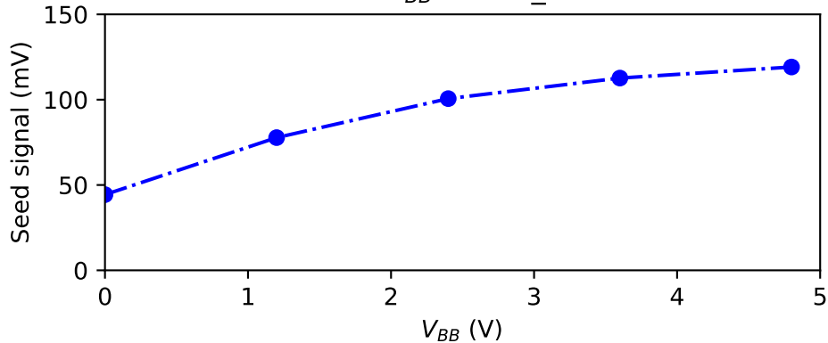
Seed VS V_{BB} AF15P_W22B32
