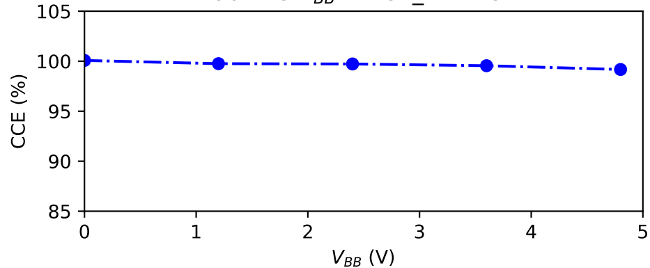
CCE VS V_{BB} AF15P_W22B32
