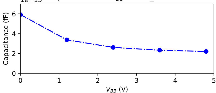
Capacitance VS V_{BB} AF15P_W22B32
